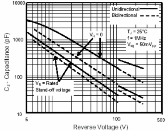
Fig. 6 - Capacitance
